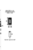
ARMAÇÃO POSITIVA DAS LAJES DO PAVIMENTO PAV. TÉRREO (EIXO Y)
